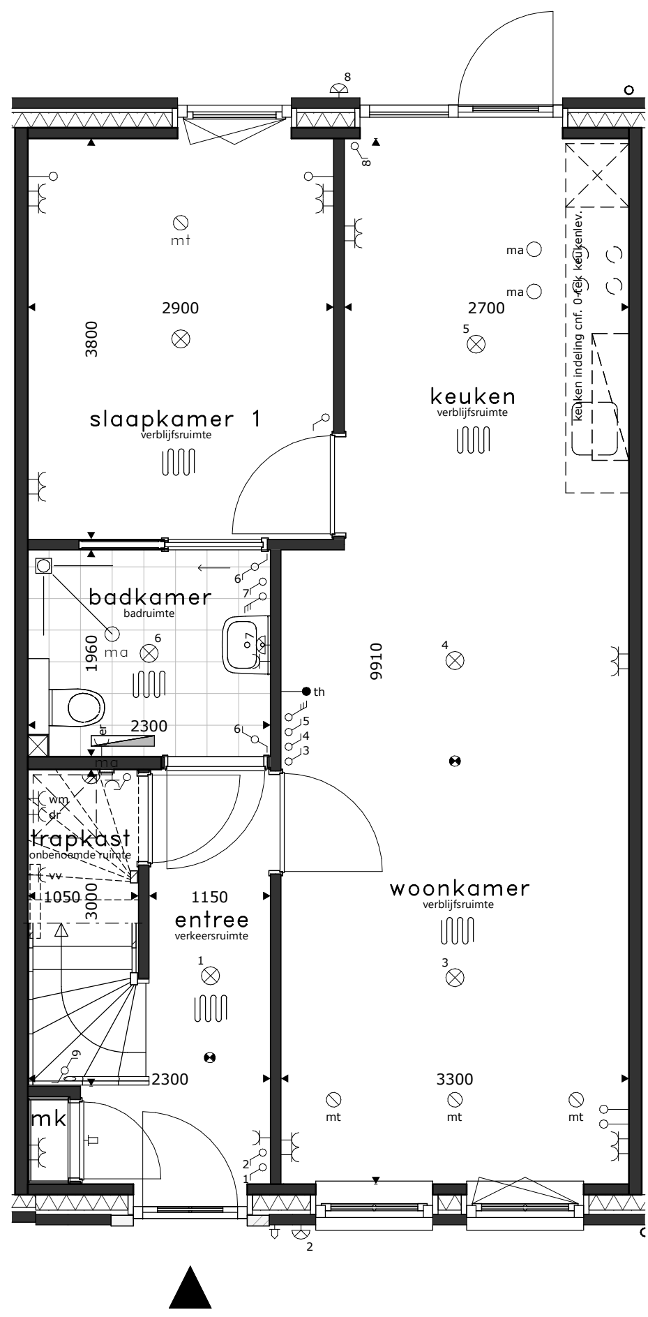
begane grond
