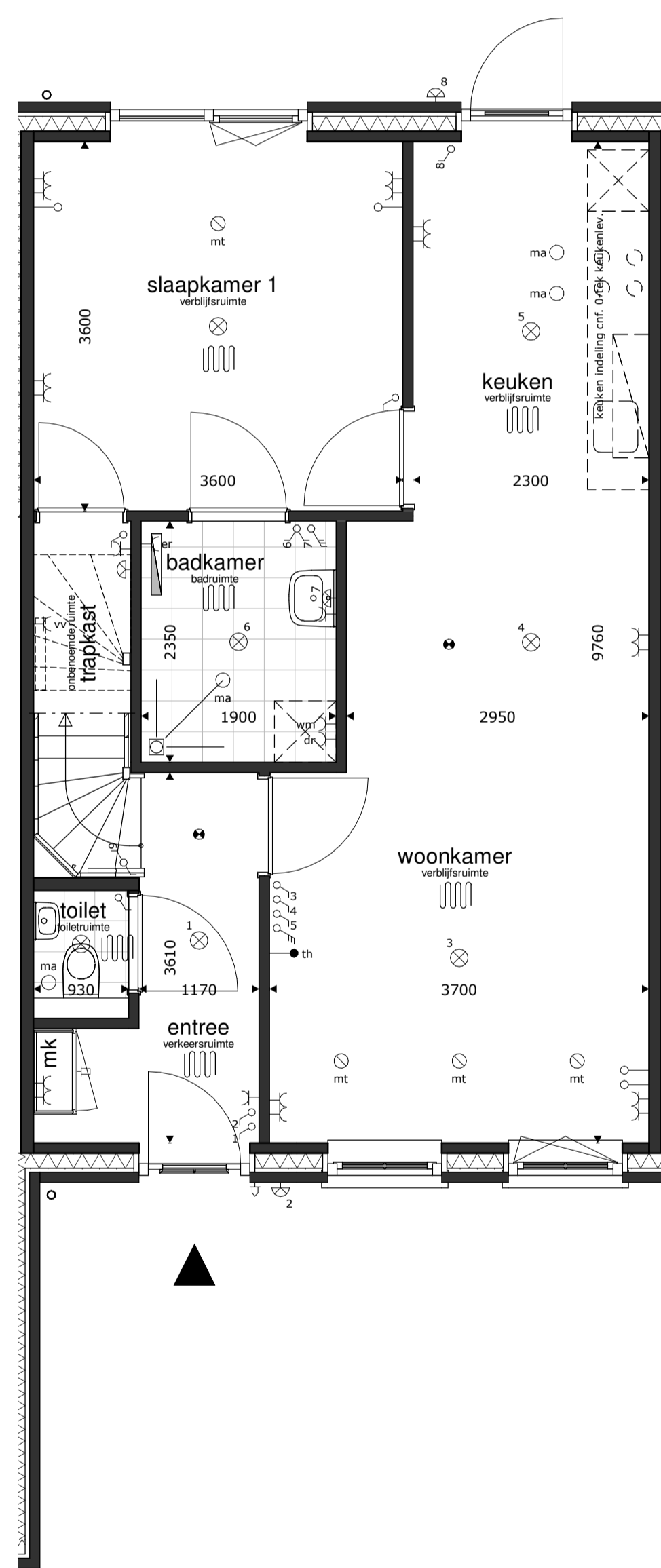
begane grond
